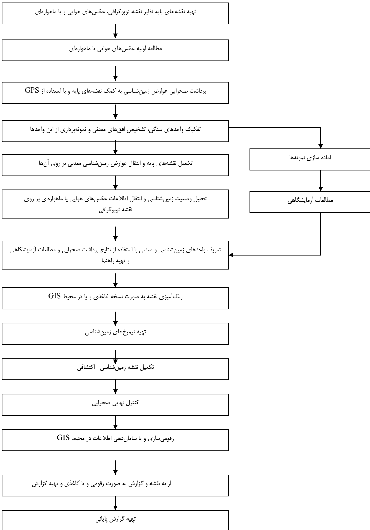
شکل ۱-۱- نمودار جریانی مراحل تهیه نقشه زمین‌شناسی اکتشافی با مقیاس ۱:۲۵,۰۰۰ و ۱:۲۰,۰۰۰
